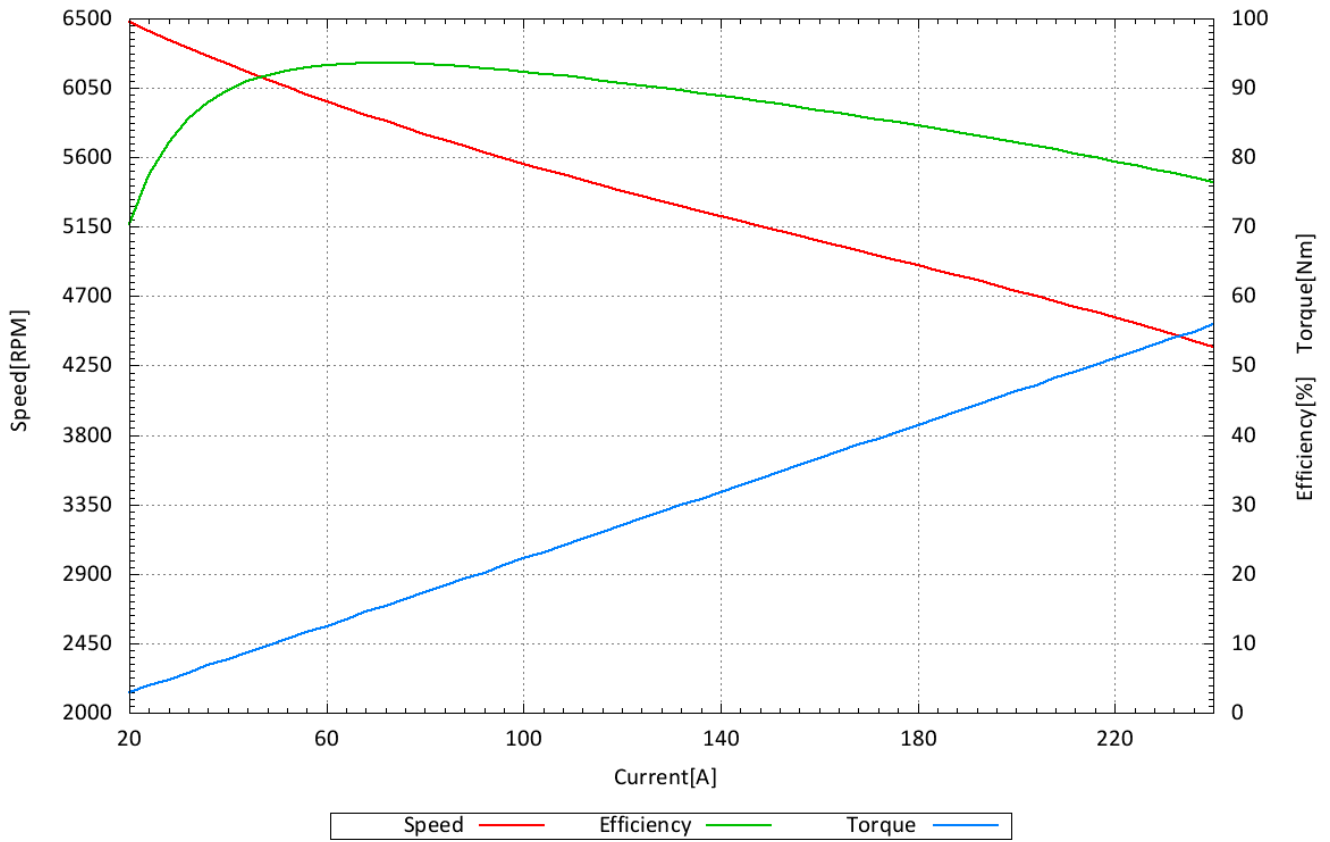
HP875_70_B6_P30_140V_MST140-200_K_09082024
