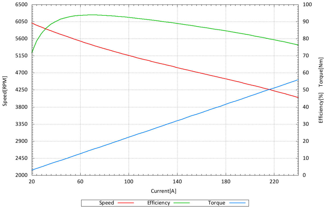
HP875_70_B6_P30_130V_MST140-200_K_09082024
