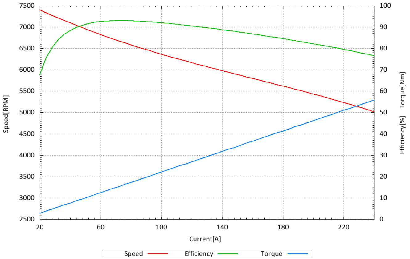
HP875_70_B6_P30_160V_MST140-200_K_09082024
