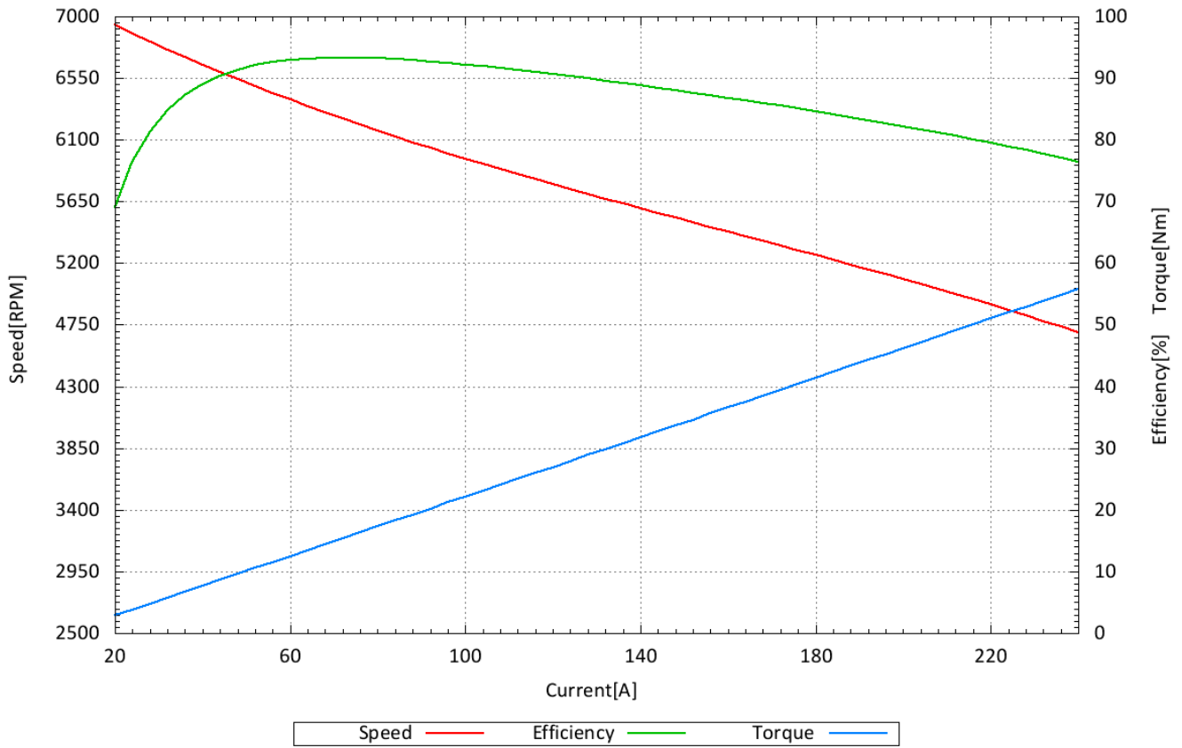
HP875_70_B6_P30_150V_MST140-200_K_09082024
